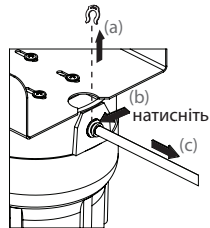
Від'єднання трубок
